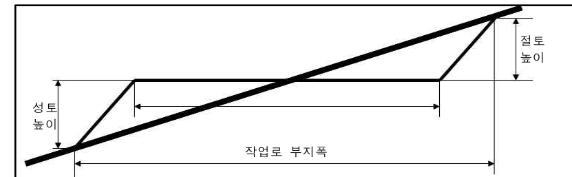
<작업로의 단면형태>
